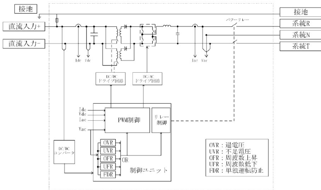
図3 BDM-300-210JD 回路図
